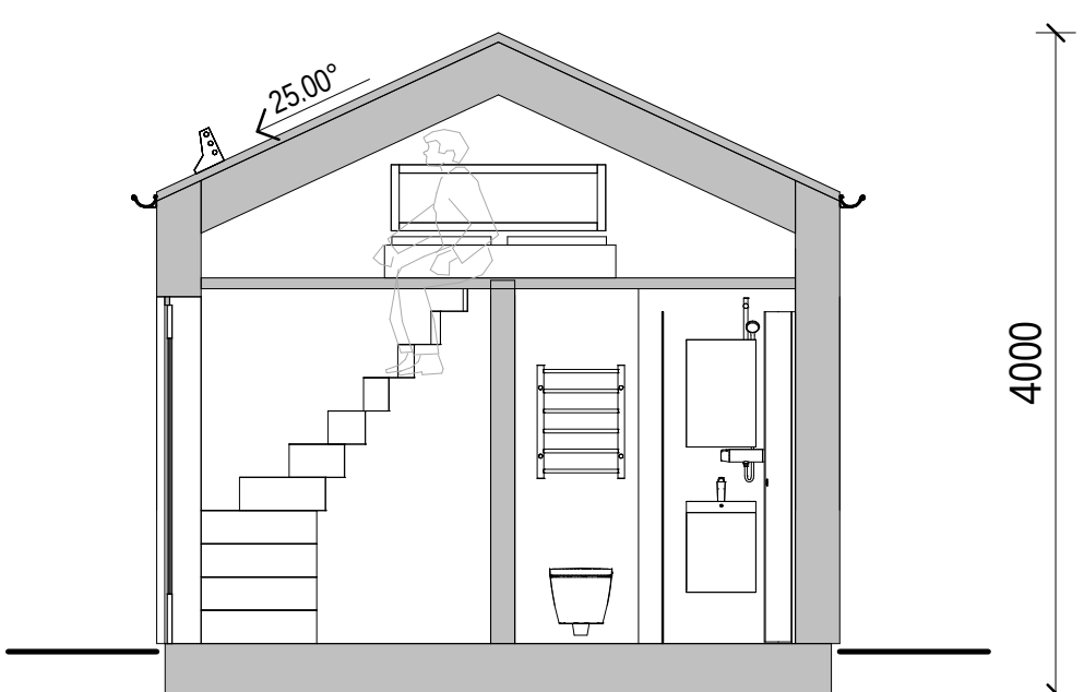
SEKTION A-A
